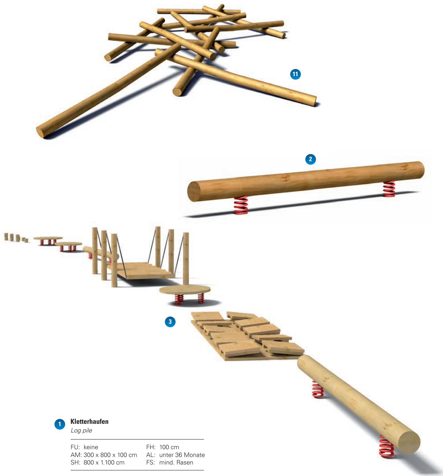
2 Wippbalken Seesaw beam FU: 2 Stück FH: 40 cm AM: 400 x 20 x 40 cm AL: über 36 Monate SH: 600 x 340 cm FS: mind. Rasen
